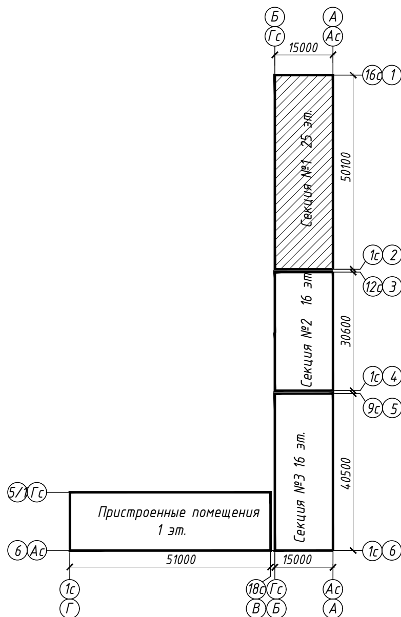
Схема блокировки
