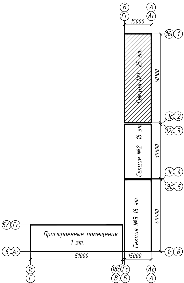
Схема блокировки
